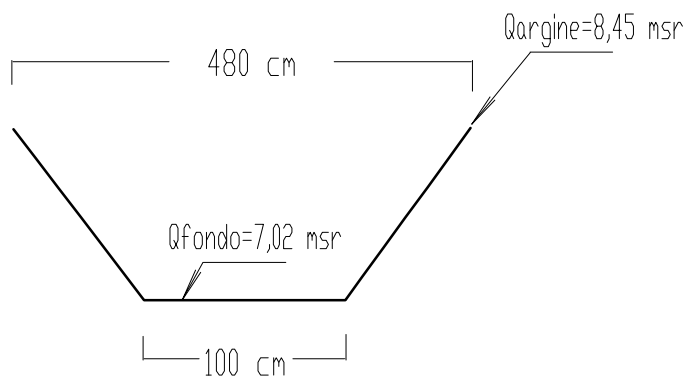
SEZIONE S032 (fuori scala)
