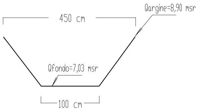
SEZIONE S013 (fuori scala)
