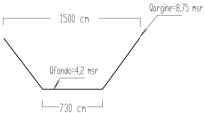
SEZIONE S055 (fuori scala)
