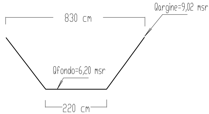
SEZIONE S030 (fuori scala)
