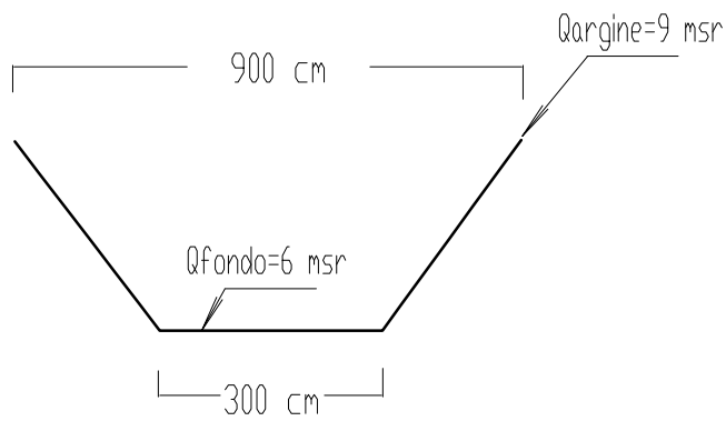
SEZIONE S043 (fuori scala)
