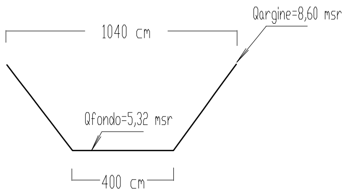
SEZIONE S036 (fuori scala)
