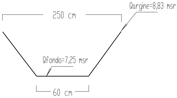
SEZIONE S001 (fuori scala)
