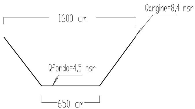
SEZIONE S044 (fuori scala)
