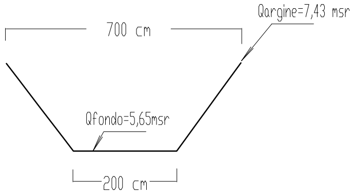
SEZIONE S046 (fuori scala)
