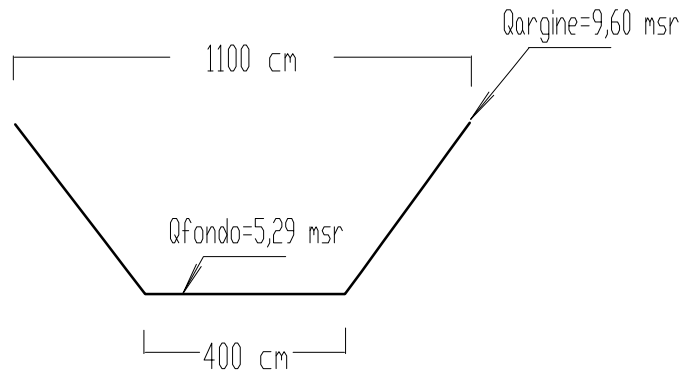
SEZIONE S018 (fuori scala)
