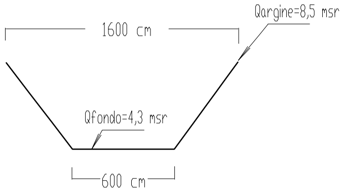
SEZIONE S050 (fuori scala)
