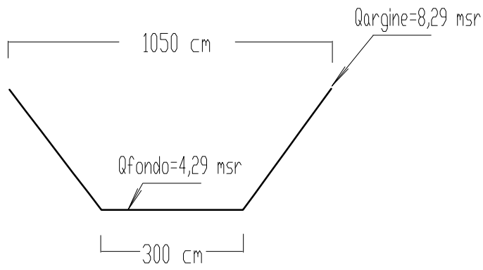
SEZIONE S061 (fuori scala)
