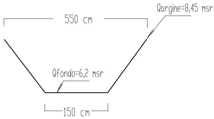
SEZIONE S041 (fuori scala)
