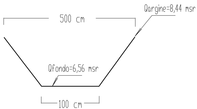
SEZIONE S040 (fuori scala)
