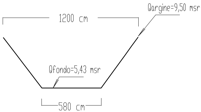
SEZIONE S023 (fuori scala)
