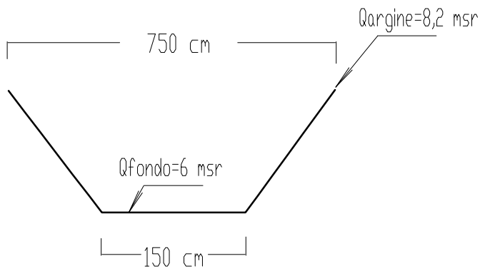
SEZIONE S047 (fuori scala)
