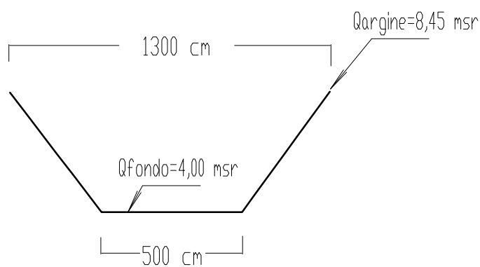
SEZIONE S060 (fuori scala)
