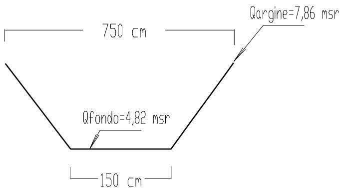
SEZIONE S054 (fuori scala)
