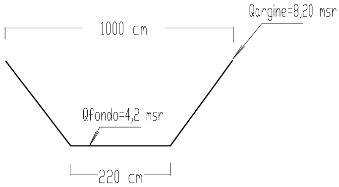
SEZIONE S062 (fuori scala)
