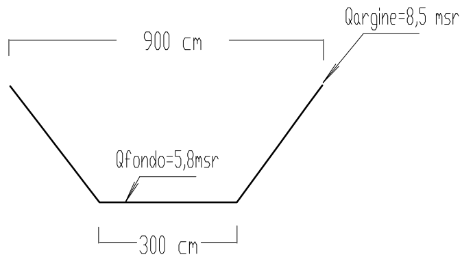
SEZIONE S042 (fuori scala)
