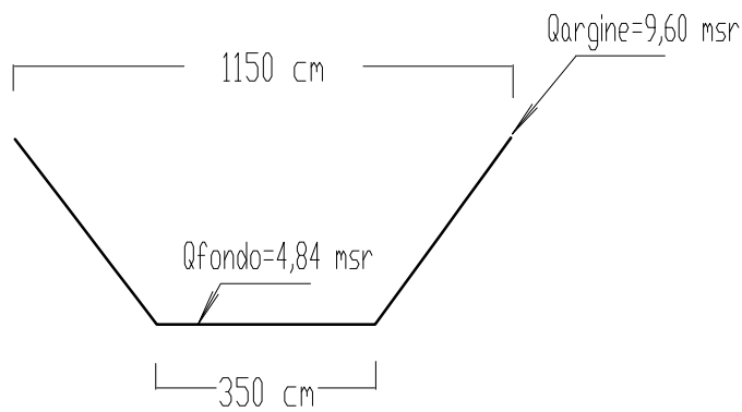
SEZIONE S019 (fuori scala)
