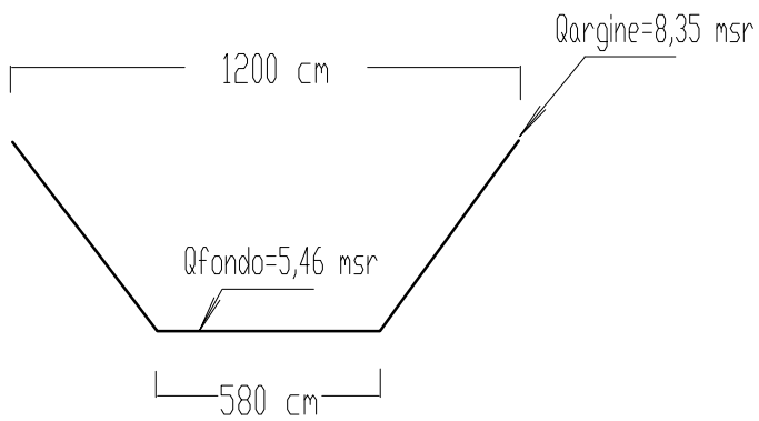
SEZIONE S024 (fuori scala)
