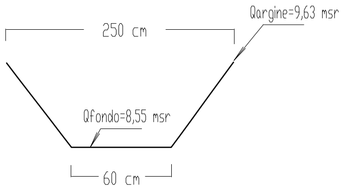
SEZIONE S005 (fuori scala)
