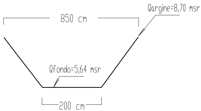
SEZIONE S035 (fuori scala)
